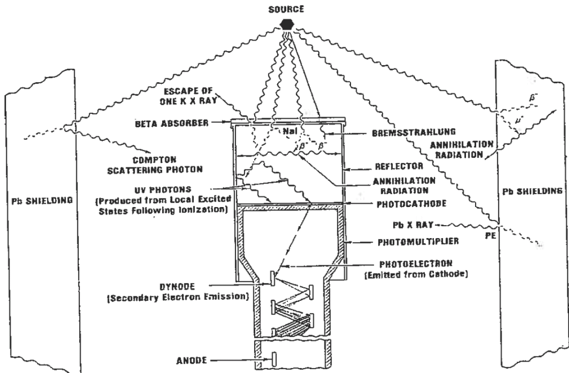
Joonis nr. 2 Gamma sähvatuste registreeria (muundur)
