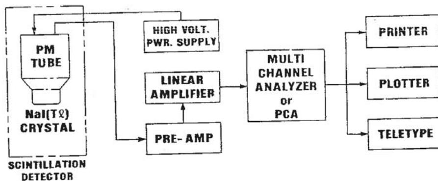
Joonis nr. 1 Gamma spektromeetri plokk skeem
